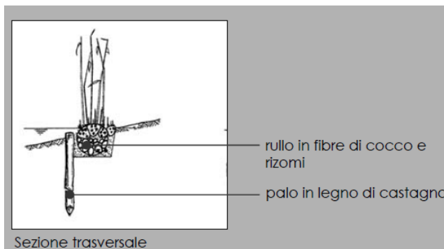
Esempio di impianto di canneto con rullo in fibre di cocco
