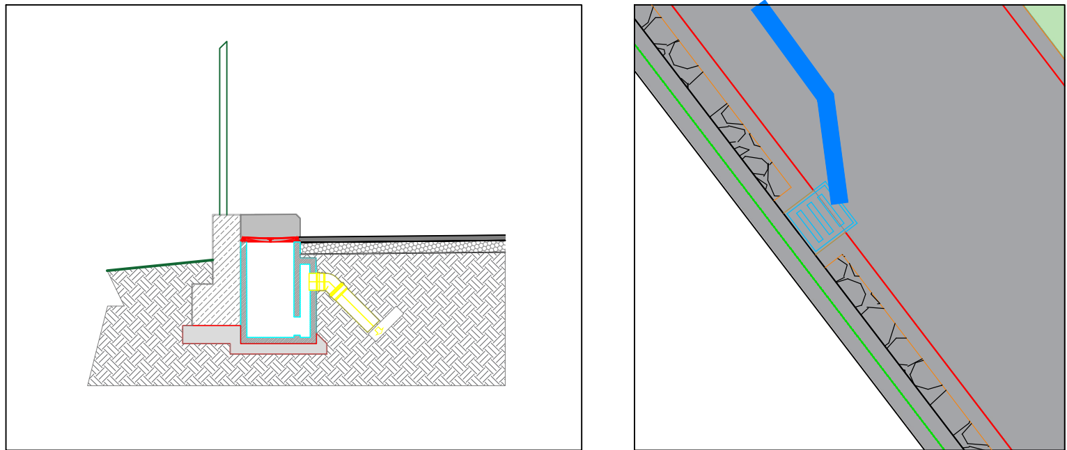
Particolare caditoie Tratti A e C
